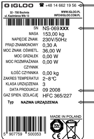
Abb.13 Typenschild
