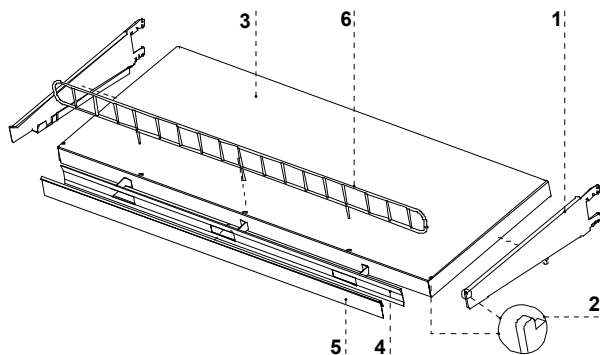
Abb.5 Regalfachsatz
