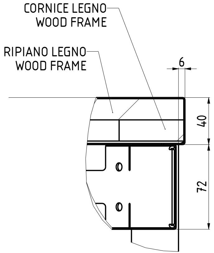
A 1:2
