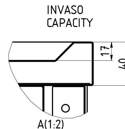
A(1:2)
