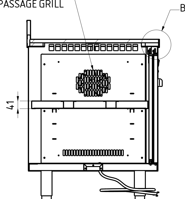
PASSAGGIO ARIA CALDA HOT AIR PASSAGE GRILL
