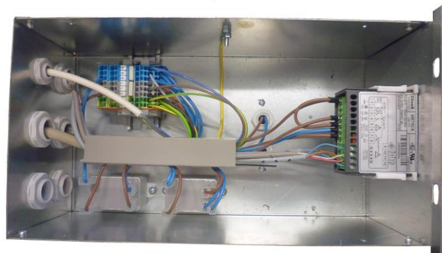
Abb. 2.4.2 - Verteilerkasten
