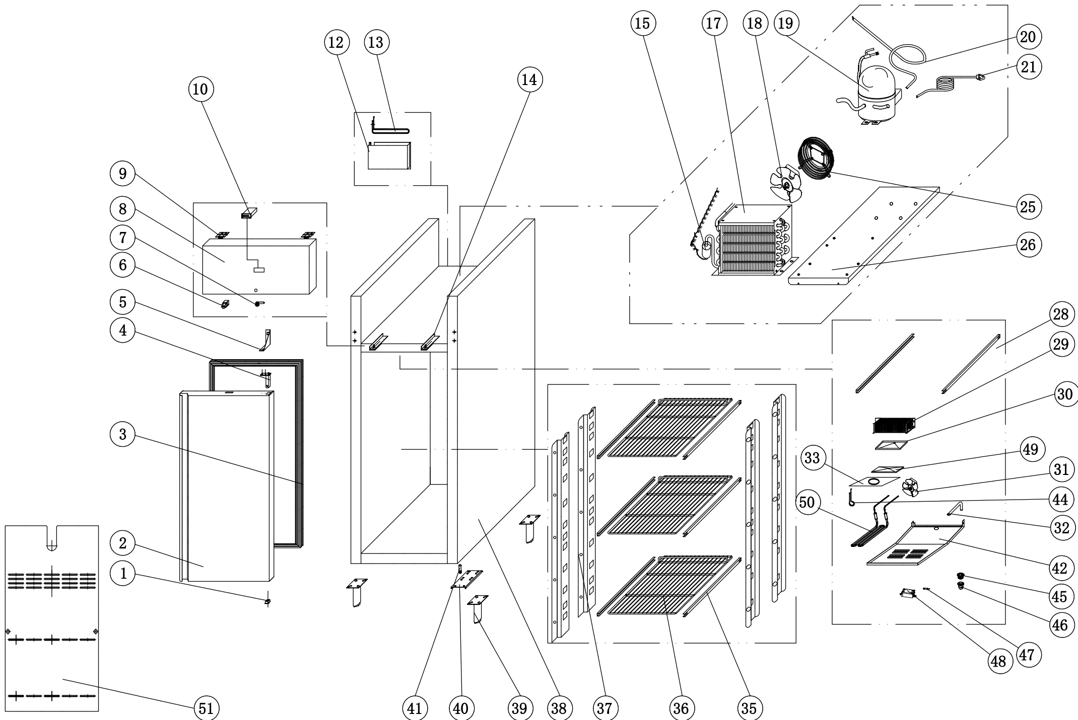
EXPLODE OF HC-GN351BT
