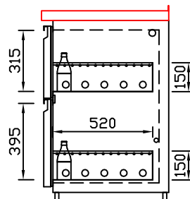
EZ-31/39 Doppelauszug 1/3-2/3 Best.-Nr.: 30110
