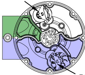
Regenerationsgetriebe
