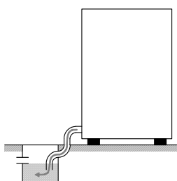
Vapaa poisto
