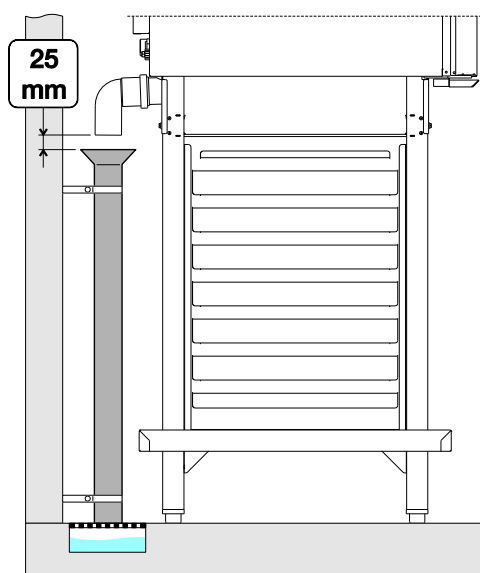
Abb. 4 Bodenanschluss auf Gitterrost
