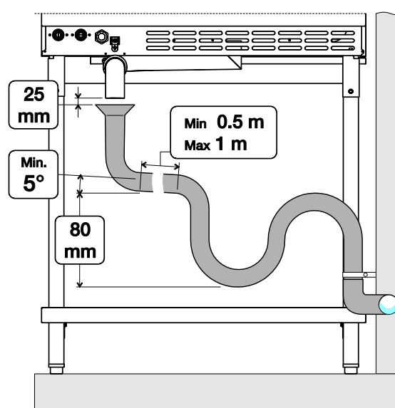
Abb. 5 Anschluss mittels Siphon
